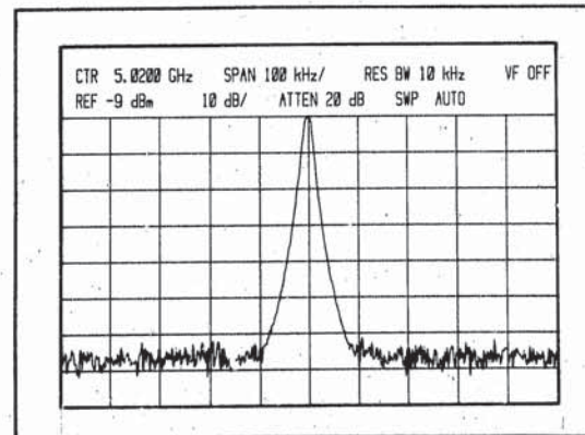
Figure 8. PER DIV Mode
