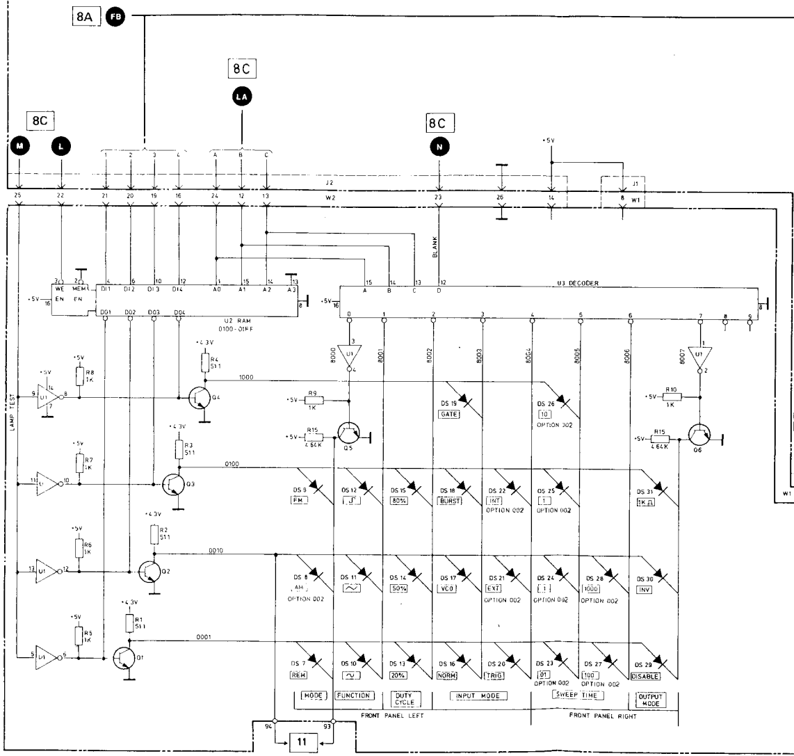
P/O A2 BD AY DISPLAY 08165-66502/19
