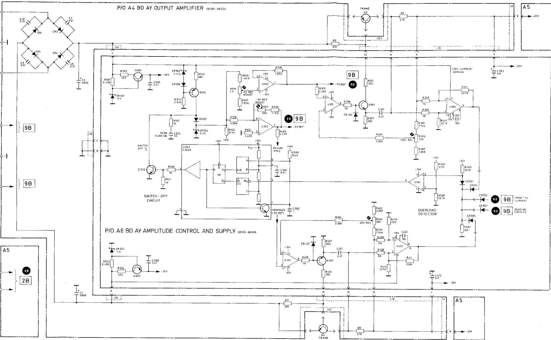
FRAME A4, A6 ± 20V SUPPLIES
