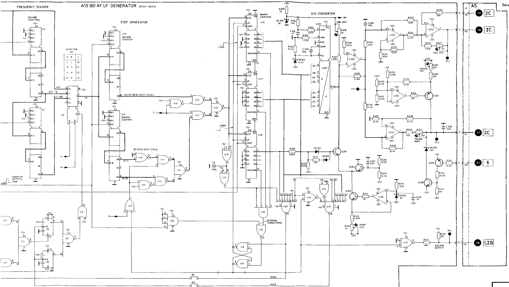
A10 LF GENERATOR
