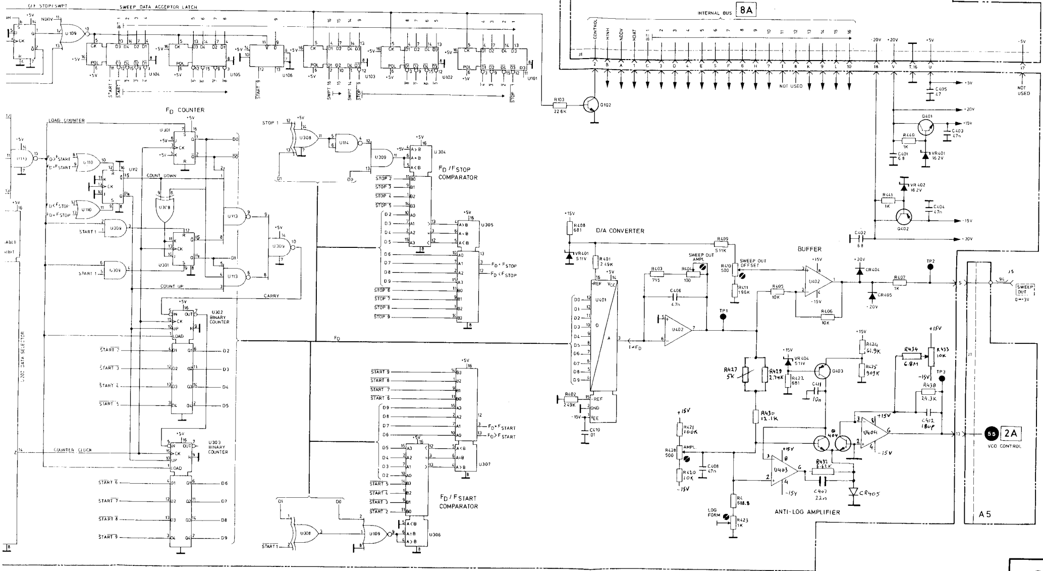
A11 SWEEP GENERATOR
