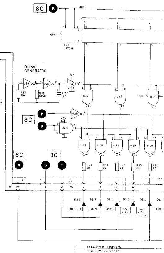
P/O A2 BD AY DISPLAY 08165-66502/19
